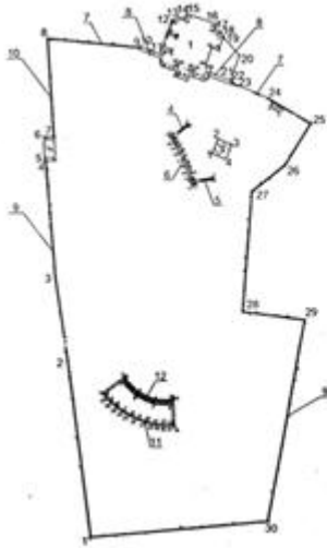
Նկ. 1. Պատվո բլուրի և մատուռի այսօրվա հատակագիծը, մասշտաբ 1:1000:
